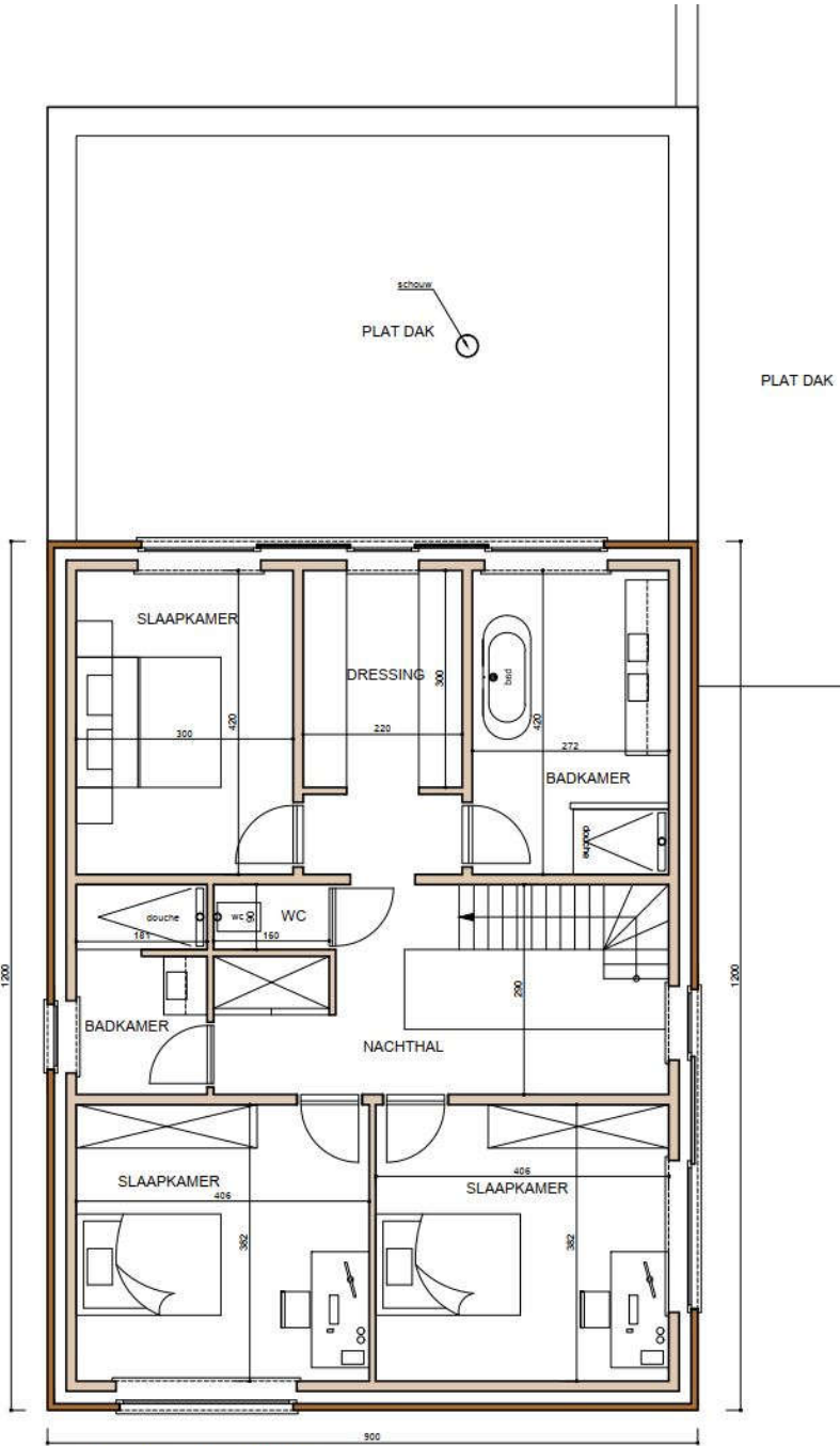
1°VERDIEPING
