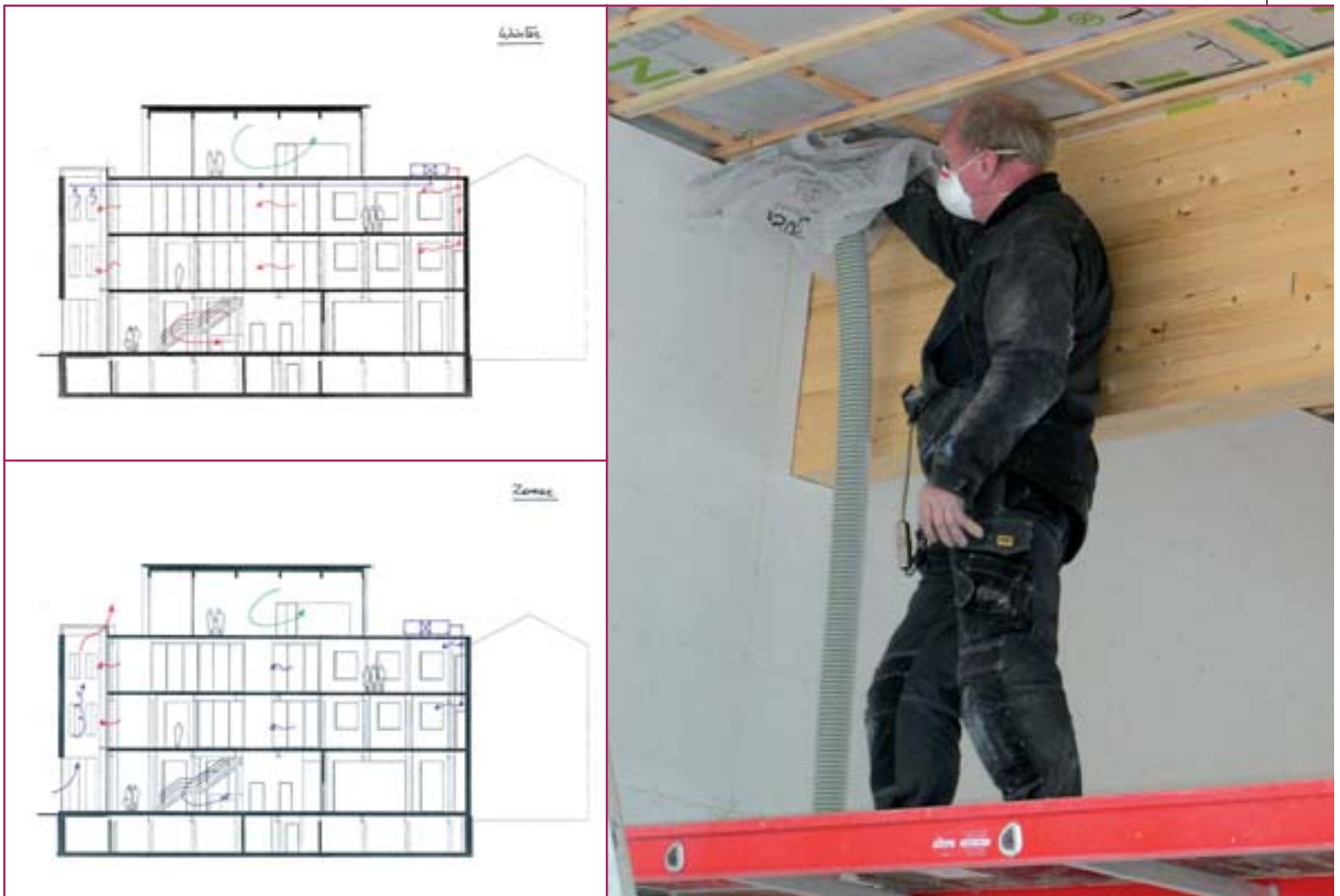
Het houten dakgebouw is geïsoleerd met papiervlokken die in het dak en de wanden werden geblazen. (Foto: Jenny Dedoncker). Op de tekeningen zie je de ventilatiestromen. Blauw is koud, rood is warm. (Tekeningen: IRS Studiebureau ir. B. Depré)
