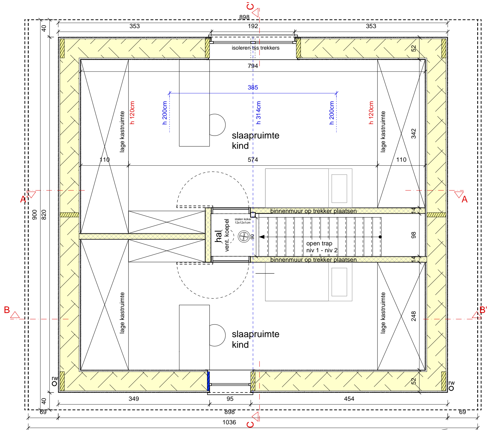
VERDIEPING 2 (zolder)
