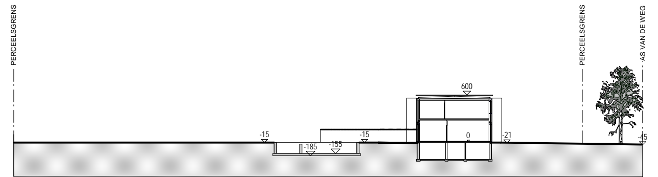
TERREINSNEDE BB 1/500
